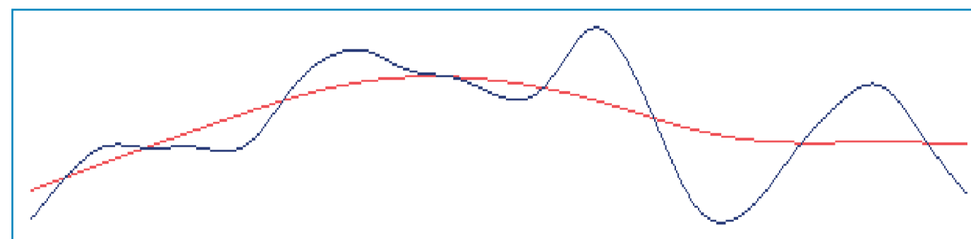
Bild 3: Lågpassfilterad medellinje från primärprofilen och medellinjen för \lambda_c -profilfilter
