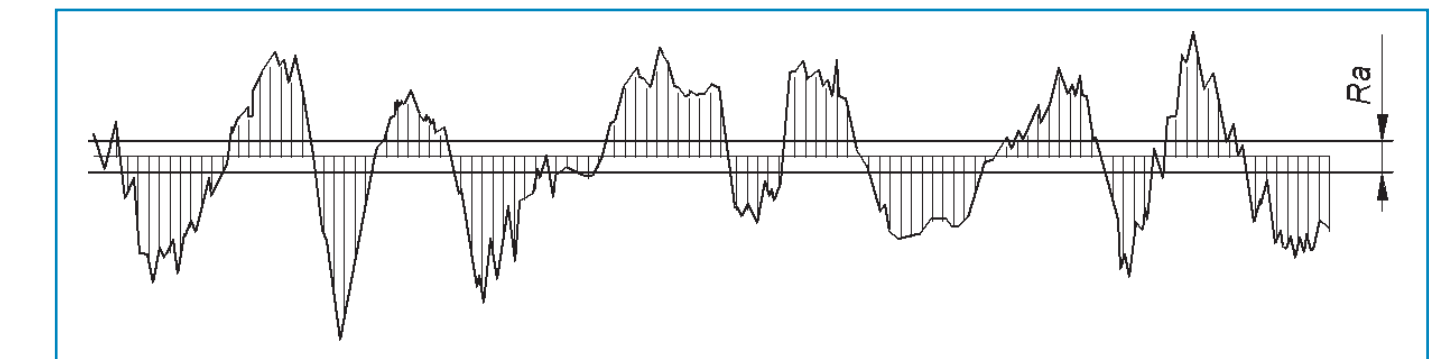
Bild 6: Profilens aritmetiska medelvärde Ra
