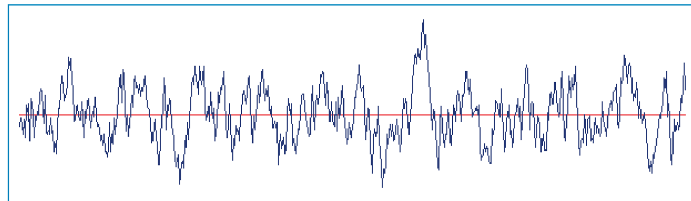
Bild 2: Ytjämnhetsprofil med medellinje (högpassfiltrering av primärprofilen med \lambda_c -profilfilter)
