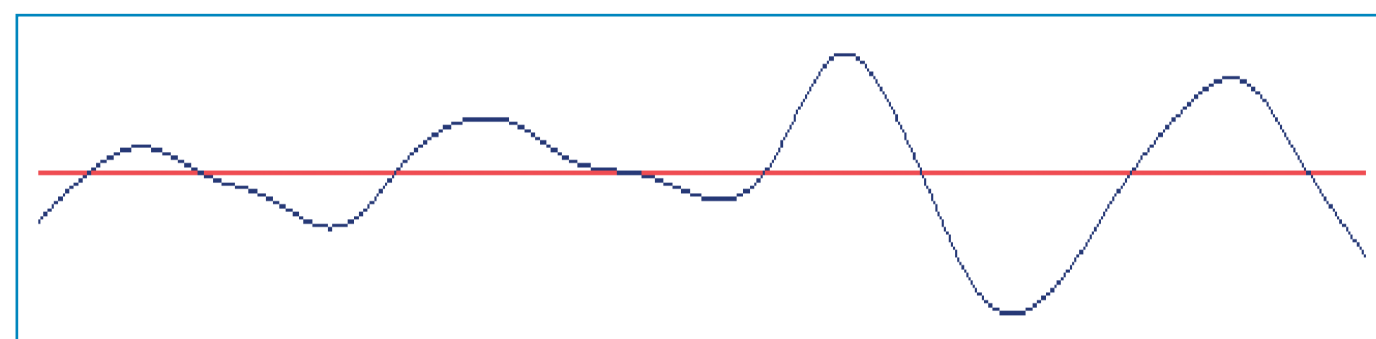
Bild 4: Vågighetsprofil med medellinje (högpassfiltrering av primärprofilen med \lambda_s -profilfilter)
