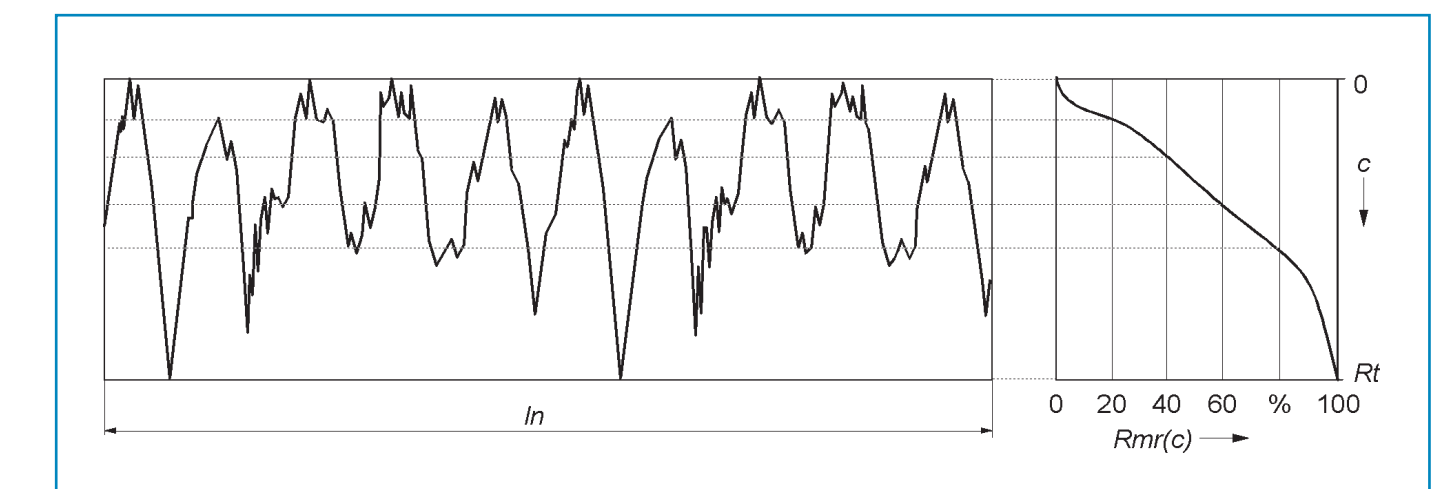
Bild 9: Profilens materialandelskurva representerande profilens materialandel Rmr(c) som funktion av nivån c (Abbott-Firestone-kurva)
