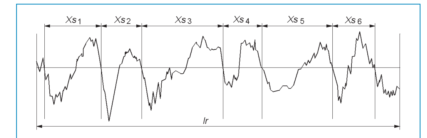
Bild 8: Profilelementens medelbredd RSm är medelvärdet av profilelementens bredder Xs
